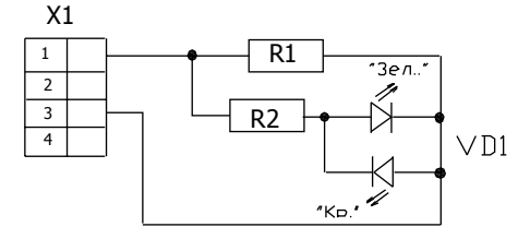
Схема электрическая
