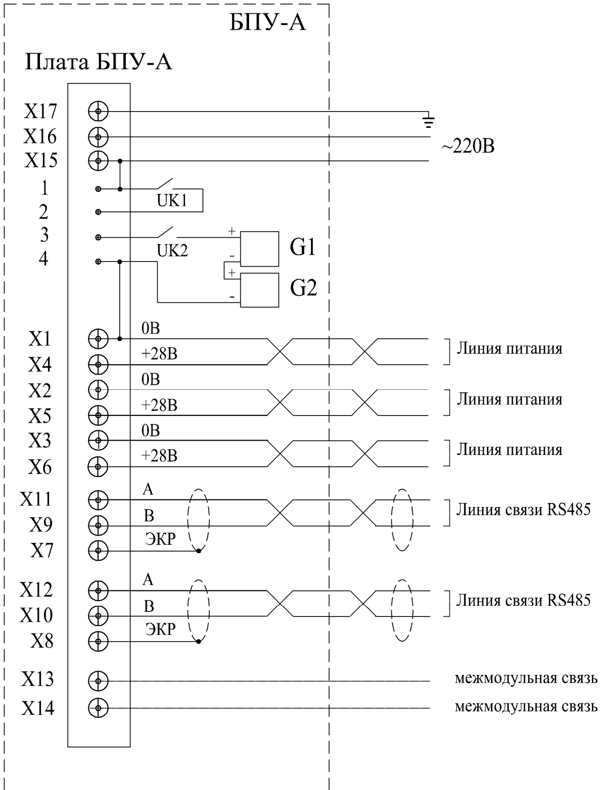
Рисунок 2. Схема подключения БПУ-А
