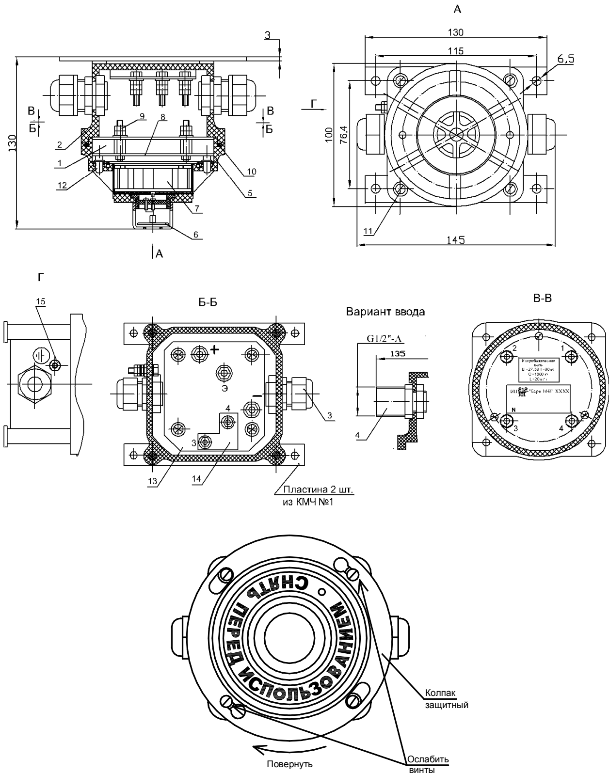
Рисунок Б.1. – Извещатель пожарный комбинированный искробезопасный ИП212/101 – "Барк М-И" Общий вид. Габаритные и установочные размеры. Крепление извещателя пластинами.
